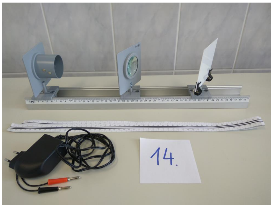
14. ábra A 14. tétel kísérleti eszközei
