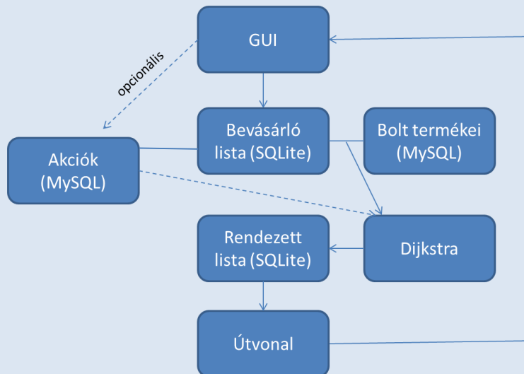
Alkalmazás működése
