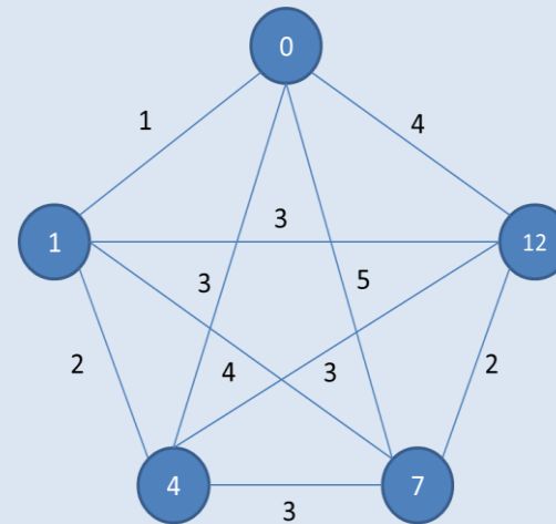
Útvonaltervezés gráffal
