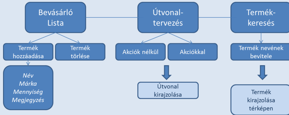
Alkalmazás működése
